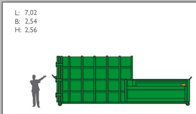
Abrollcontainer mit Presse 20 m 3
